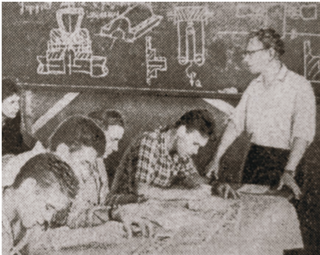
На данной фотоснимке – процесс обучения рабочих, которые будут осваивать седьмую бумагоделательную машину. Бумажники внимательно слушают объяснения старшего инженера-конструктора Ю.А. Артемьева. Тема занятия – устройство рулонного крана. 1965 год
