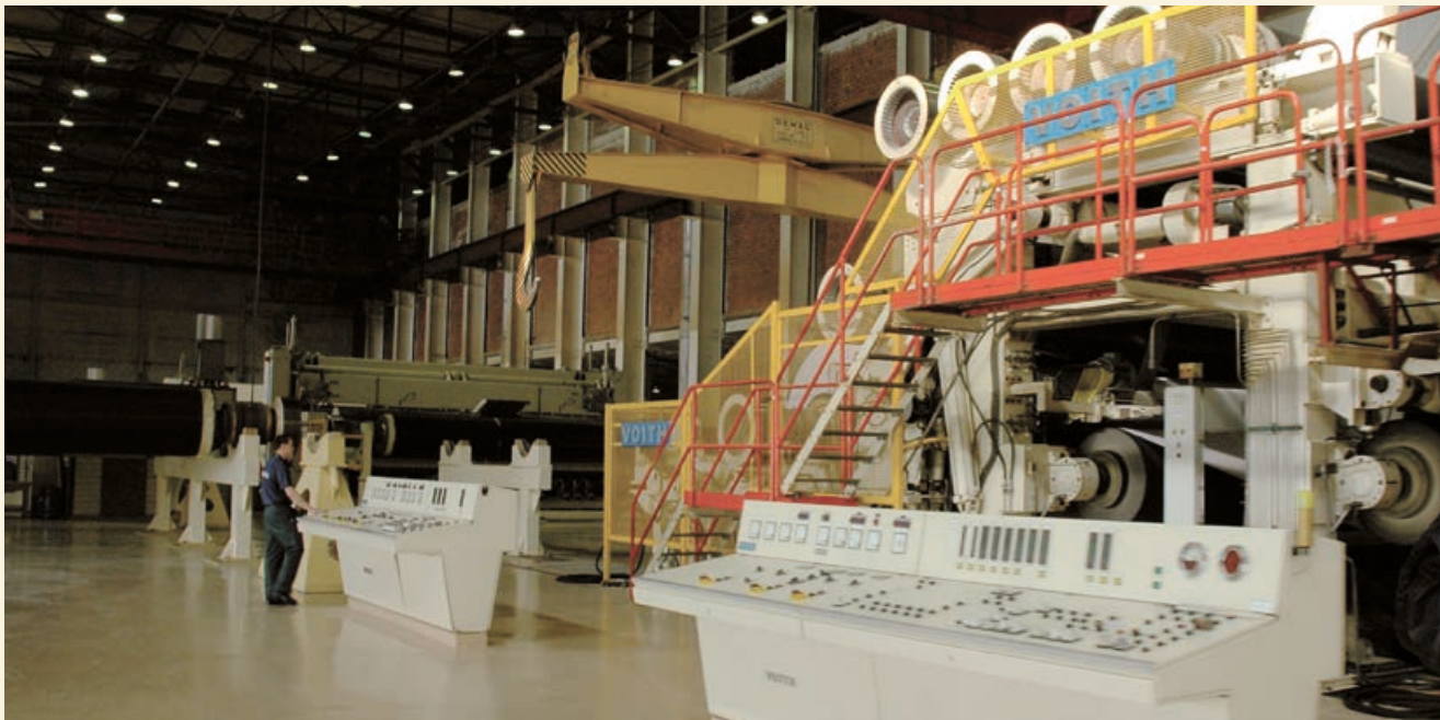
Бумагоделательная машина №8 является уникальной не только для нашей страны, но и для Европы как по ее быстроходности, так и по возможности производить высококачественную продукцию.
